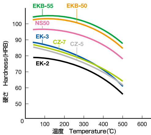
高温硬さ High temperature hardness
