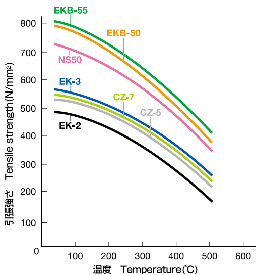
高温強度 High temperature strength
